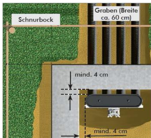
Bild 3: Platzierung Rohbauteil
