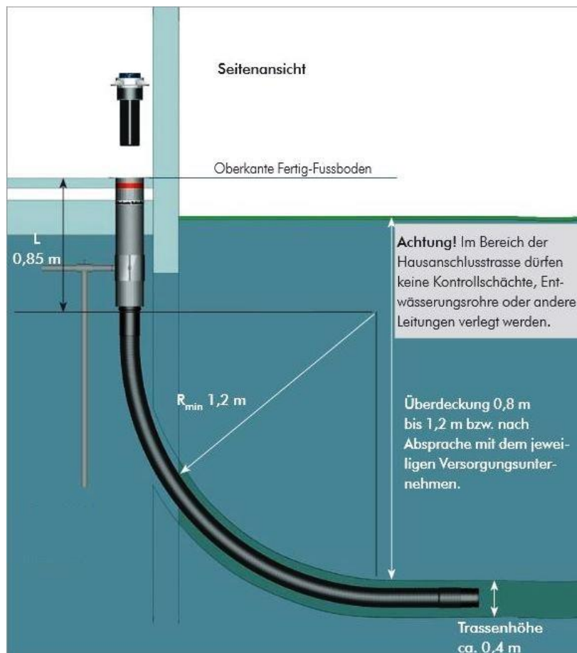
Bild 1: Seitenansicht Rohbauteil
